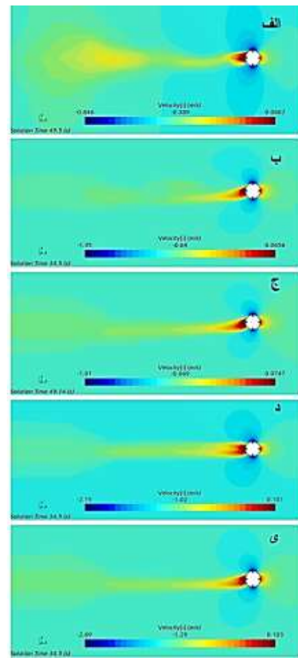
شکل ۱۴. توزیع سرعت در راستای محور X و عمق ۲/۷ متری از سطح آب و (الف) سرعت ۰/۵ متر بر ثانیه جریان ب) سرعت ۰/۷۵ متر بر ثانیه جریان ج) سرعت ۱/۰۰ متر بر ثانیه جریان د) سرعت ۱/۲۵ متر بر ثانیه جریان ی) سرعت ۱/۵ متر بر ثانیه جریان
