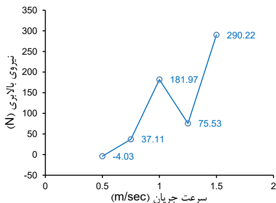
شکل ۱۱. تغییرات نیروی بالابری کل سازه بر حسب سرعت‌های مختلف جریان
