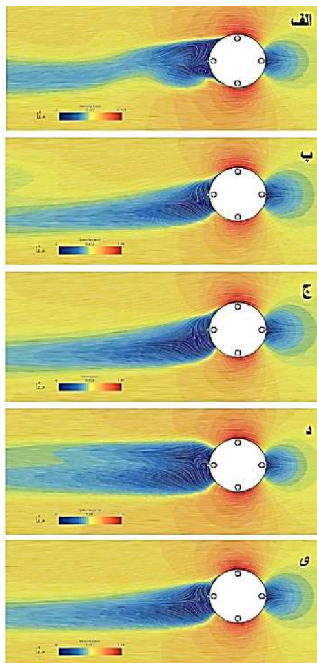
شکل ۱۵. توزیع بردار سرعت در اطراف سازه ریگ اسپار دارای سازه مارپیچی و در عمق ۲/۷ متری از سطح آب (الف) سرعت ۰/۵ متر بر ثانیه جریان ب) سرعت ۰/۷۵ متر بر ثانیه جریان ج) سرعت ۱/۰۰ متر بر ثانیه جریان د) سرعت ۱/۲۵ متر بر ثانیه جریان ی) سرعت ۱/۵ متر بر ثانیه جریان
