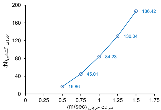
شکل ۶. تغییرات نیروی کششی قسمت بدنه استوانه ای اسپار بر حسب سرعت های مختلف جریان
