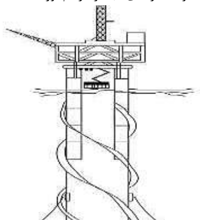
شکل ۱. نمای کلی ریگ اسپار با طوقه مارپیچی
